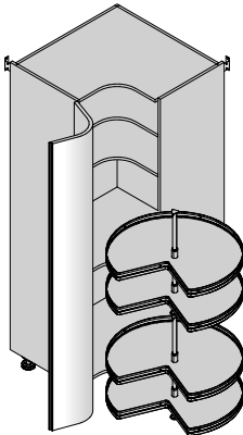
L 95 H 208 - 221 P 95
